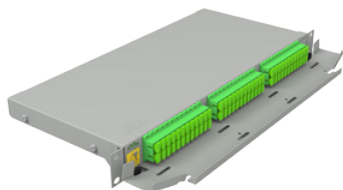
Przełącznica światłowodowa PS-19/HD 1U
