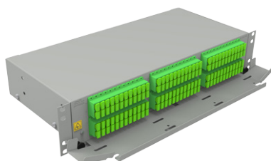
Przełącznica światłowodowa PS-19/HD 2U
