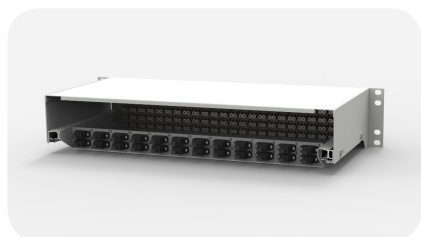
Przełącznica PS-19/288LC/2U
