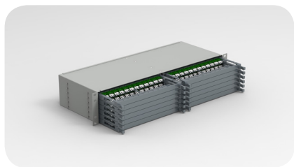
Przelącznica PNM-2
