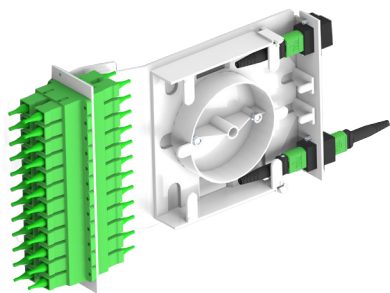
Moduł MPS-DC-2MPO/24SC-ZK
