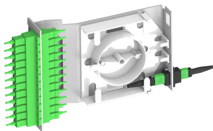
Moduł MPS-DC-2MPO/12SC-ZK
