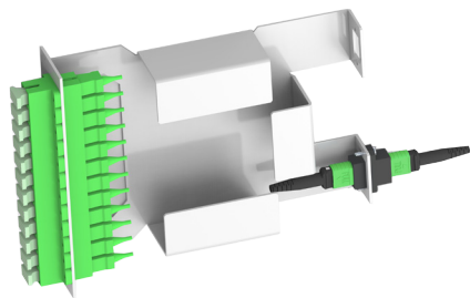
Moduł MPS-DC-2MPO/12SC-Z
