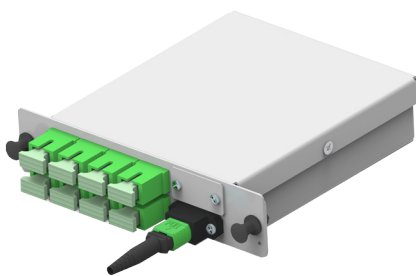
Moduł DC-LGX-8SC/2MPO
