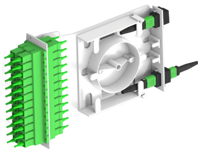
MPS-DC-2MPO/24SC-ZK Module
