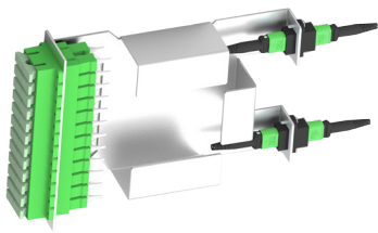
MPS-DC-2MPO/24SC-Z Module
