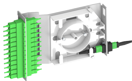
MPS-DC-2MPO/12SC-ZK Module
