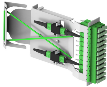
MPS-DC-2MPO/24SC Module
