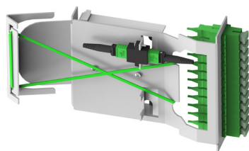
MPS-DC-2MPO/12SC Module
