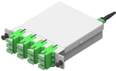
DC-LGX-12SC-2MPO Module
