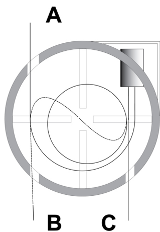
Zasobnik światłowodowy ZK-1
